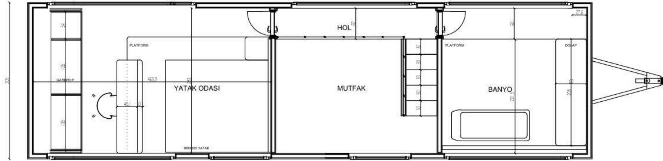
ÜST KAT PLAN GÖRÜNÜŞ B-B KESİTİ
