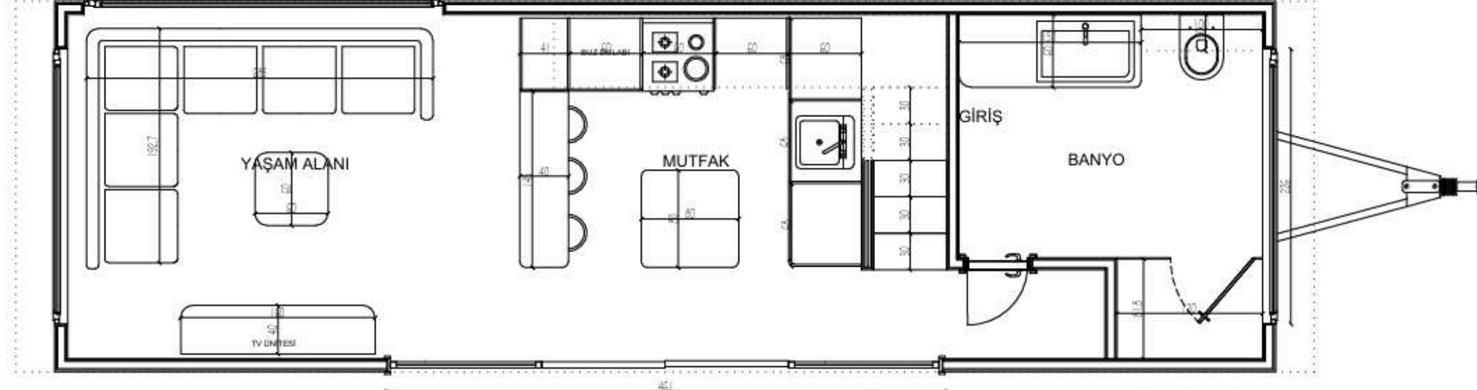
ZEMİN KAT PLAN GÖRÜNÜŞ
