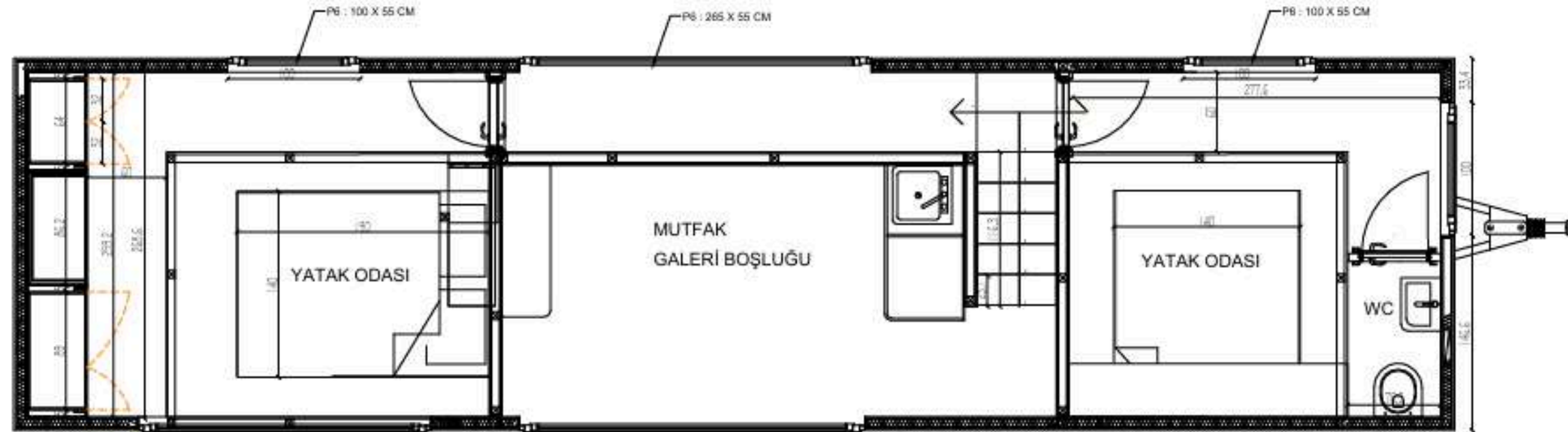
ZEMİN KAT PLANI
